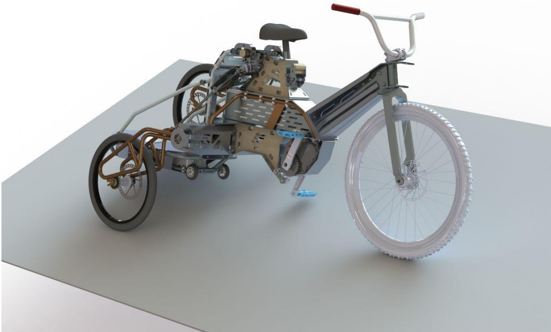
Vue 3D Solidworks
